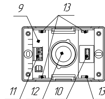
Вид спереди со снятой передней панелью
