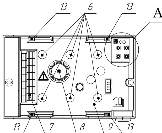
Вид спереди со снятой передней панелью
